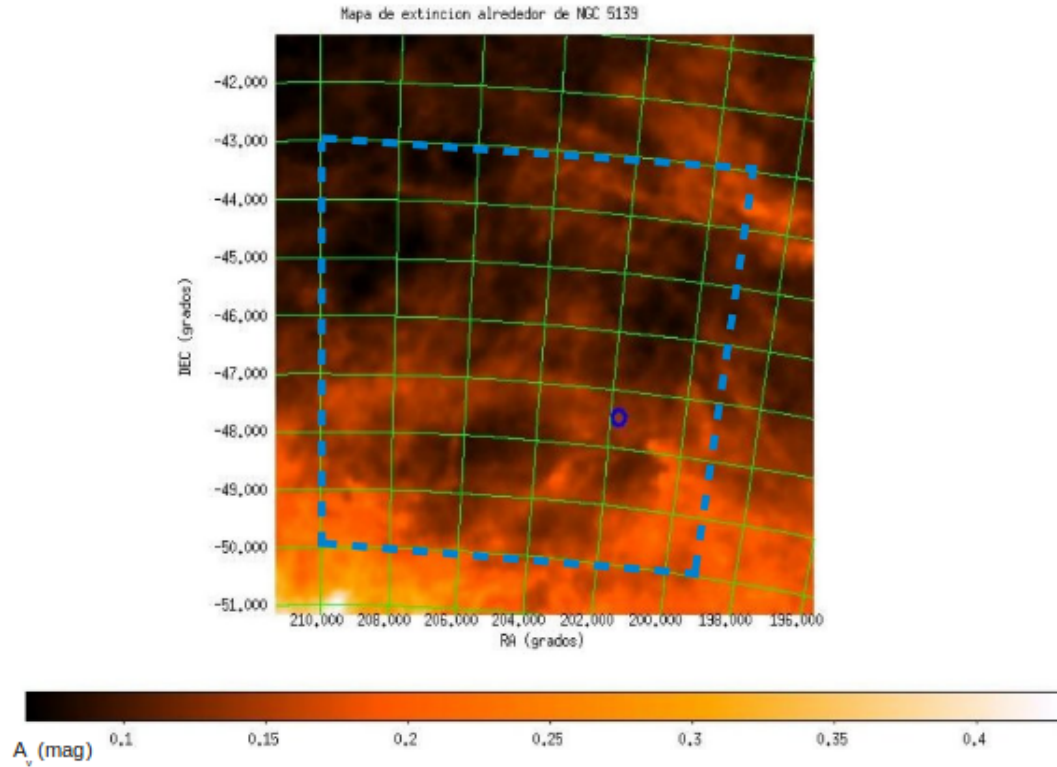
Figura 5.6: Mapa de extinción alrededor de NGC5139. El polígono de color azul es la región observada por el Telescopio Schmidt (CIDA). La circunferencia de color azul representa las coordenadas centrales de NGC5139.
