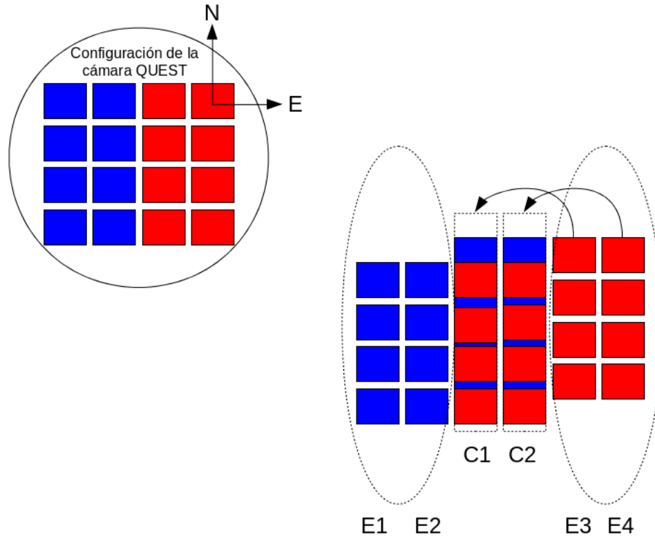
Figura 3.3: Ejemplo de la configuración de las observaciones realizadas con el telescopio Jürgen Stock. Extremo superior izquierdo, el arreglo de CCD de la cámara QUEST con sus respectivo juego de filtros (Rojo: Filtro I y en Azul: Filtro V). Supongamos que se quieren observar los campos C1 y C2 en los filtros I y V. La secuencia comienza desde el Este al Oeste. Inicialmente se observan los campos C1 y C2 en el filtro V. Posteriormente se mueve el telescopio de tal manera que los campos C1 y C2 sean observados con los filtros I. Todos los campos EX, X=1,2,3,4 son observados entonces en una sola banda. Sin embargo, no significa que no sean útiles para nuestro trabajo, pues se pueden obtener series de tiempo de estrellas en esa zona.
