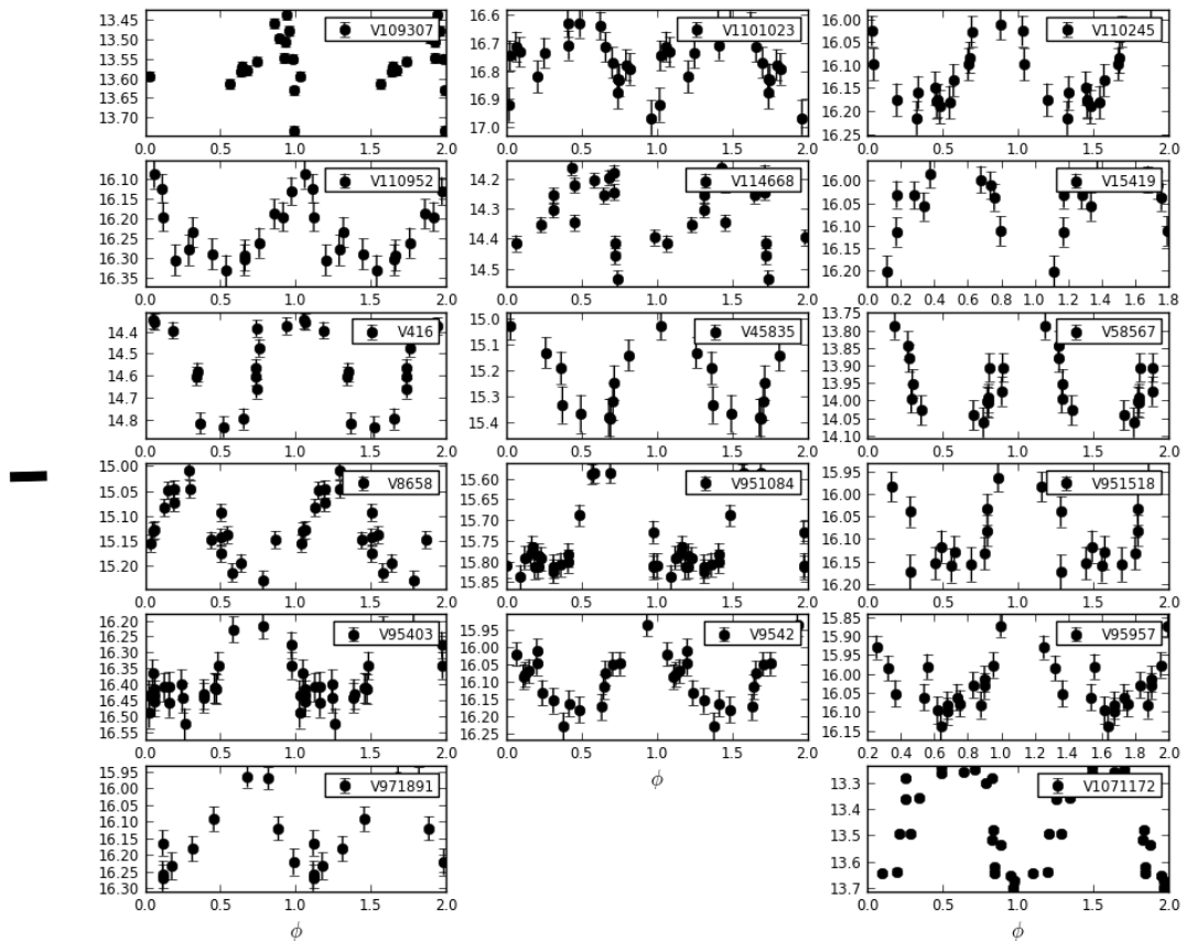
Figura 1.1: Curvas de Luz para 17 estrellas candidatas a RR Lyrae encontradas en la zona de baja completitud. El eje vertical de las curvas corresponde a las magnitudes en el filtro I.
