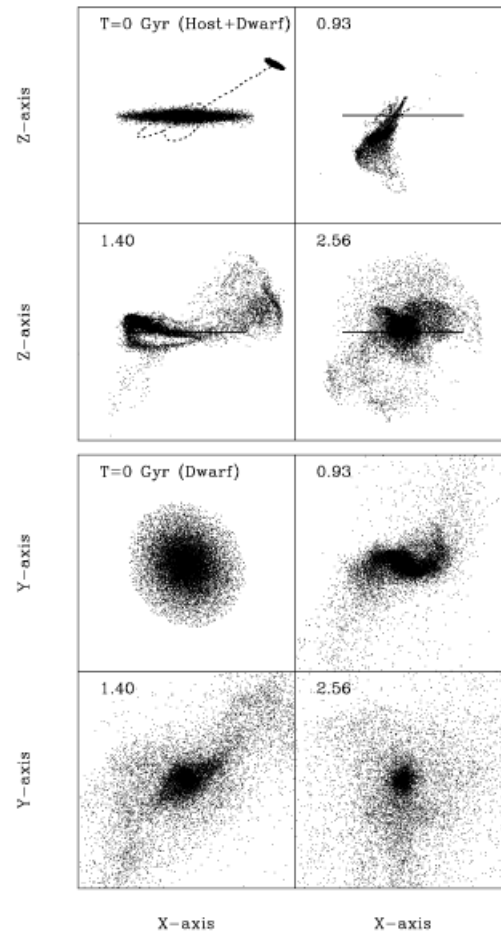
Figura 2.4: Simulación de N-cuerpos (95 mil partículas para el progenitor asociado a Omega Centauri). Tiempo de evolución del modelo de 2,56 Giga años. Los primeros 4 paneles superiores, se observa el momento antes y después del progenitor en la colisión con el disco de la Galaxia, visto en el plano (X, Z) . Y en los 4 últimos cuadros, se muestra la apariencia física del progenitor antes y después de la colisión en el plano (X, Y) . Imagen tomada de Bekki & Freeman (2003).
