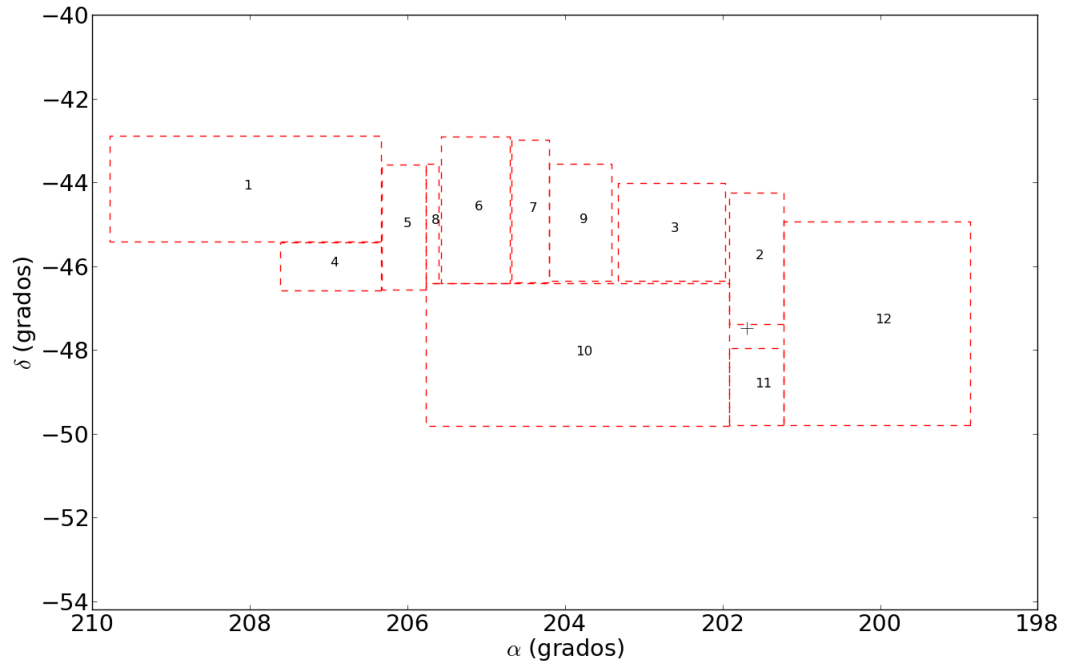
Figura 5.6: Sub-campos alrededor de Omega Centauri usadas para estimar el número esperado de estrellas RR Lyrae tanto del Halo como del Disco Grueso. El centro del cúmulo es representado con una cruz.
