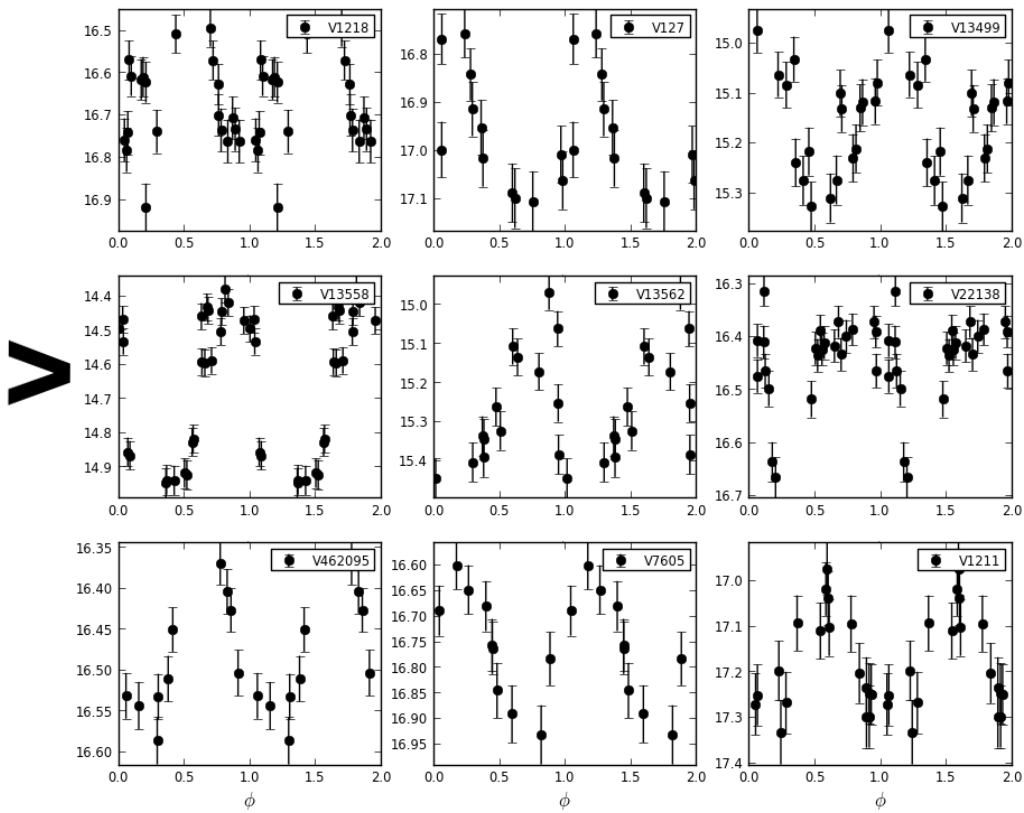
Figura 1.2: Curvas de Luz para 9 estrellas candidatas a RR Lyrae encontradas en la zona de baja completitud. El eje vertical de las curvas corresponde a las magnitudes en el filtro V.
