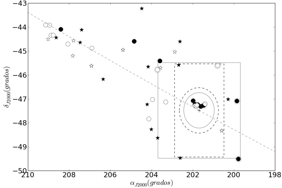
Figura 5.4: Distribución espacial de todas las estrellas RR Lyrae detectadas en el presente trabajo. La línea discontinua corresponde a una fracción de la órbita del cúmulo que se calculó a partir de sus movimientos propios (Dinescu et al. 1999). Los polígonos de líneas continuas y discontinuas, corresponden al área explorada por Leon et al. (2000) y Da Costa & Coleman (2008), respectivamente y los radios de marea asumidos por ambos autores ( r_t = 57 arcmin y r_t = 44,4 arcmin, respectivamente). Los símbolos abiertos y llenos corresponden a estrellas RR Lyrae tipo-c y tipo-ab, respectivamente. Los círculos son estrellas RR Lyrae con distancia similar a la del cúmulo ( 3,5 \text{ kpc} \leq D_\odot \leq 9,0 \text{ kpc} ) mientras que las estrellas corresponden a objetos en el campo de visión por delante ( D_\odot < 3,5 \text{ kpc} ) o por detrás del cúmulo ( D_\odot > 9,0 \text{ kpc} ). Los símbolos encerrados dentro de un círculo grande corresponden a las estrellas RR Lyrae a las cuales se les pudo hacer espectroscopía ver la sección 5.3.
