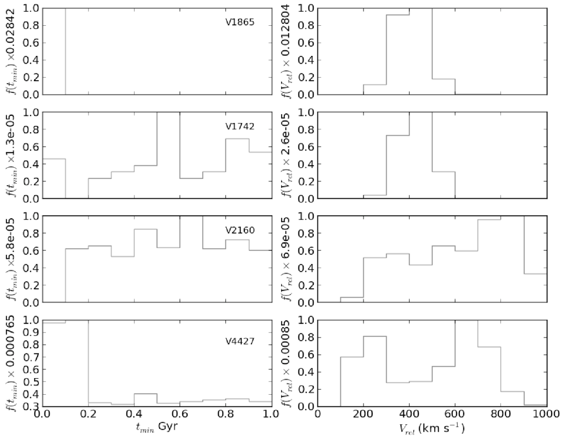
Figura 5.12: Distribución de los encuentros de los pares RR Lyrae-Omega Centauri. Izquierda: Se representa la probabilidad de encuentros ( d_{min} \leq 75\text{pc} ) en intervalos de 0,1 Giga años. Derecha: Se representa la frecuencia observada de la velocidad en el encuentro, en intervalos de 100 \text{ km s}^{-1} .
