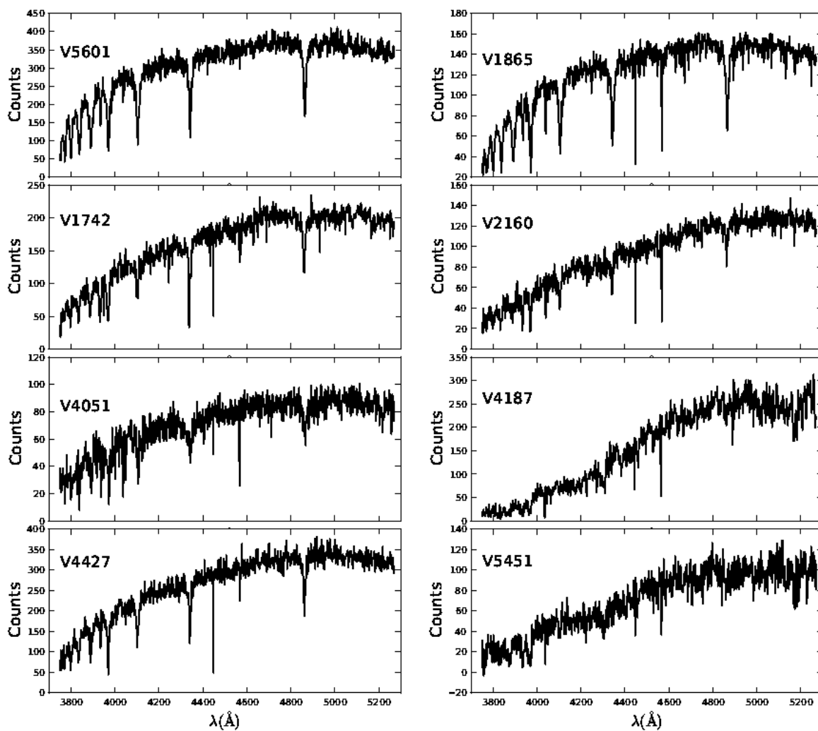
Figura 5.8: Espectros de las 8 estrellas variables RR Lyraes estudiadas.
