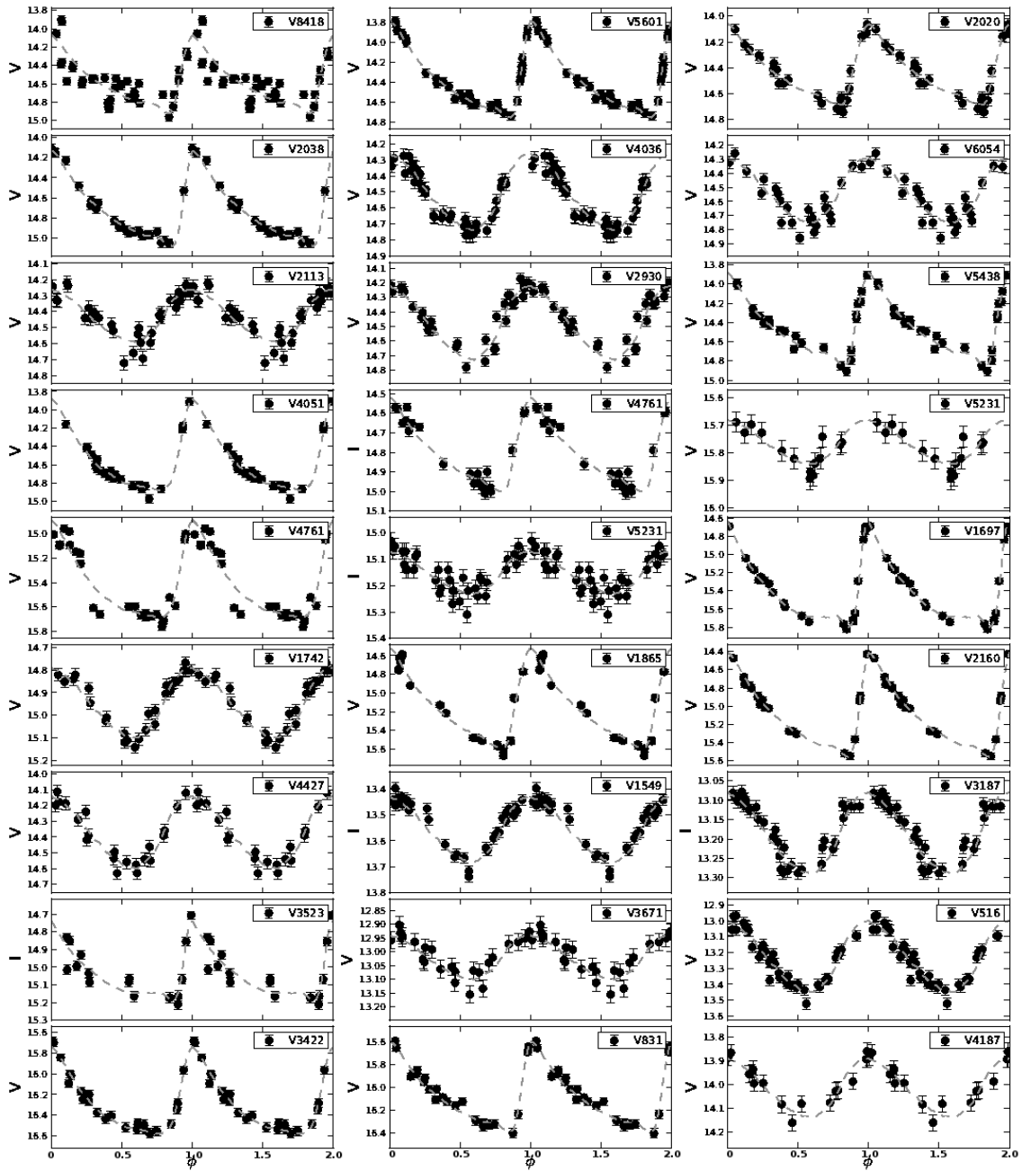
Figura 5.1: Curvas de luz de estrellas variables.
