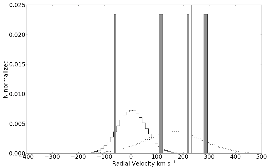
Figura 5.10: Distribución de velocidades radiales, para las 6 estrellas RR Lyrae son representadas con barras de color gris, la línea vertical delgada corresponde a la velocidad radial del cúmulo globular Omega Centauri [ V_r = 232, 2 \pm 0, 7 \text{ km s}^{-1} ; Dinescu et al. (1999)]; el histograma de línea continua representa la distribución de velocidades de estrellas del Disco, y el histograma con líneas discontinuas representa la distribución de velocidades de estrellas del Halo.
