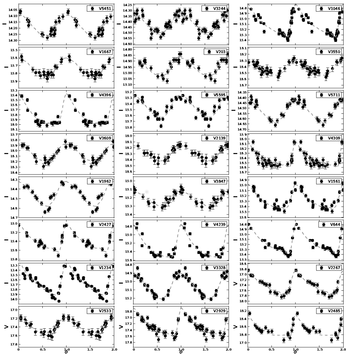
Figura 5.2: Continuación de la Figura 5.1.
