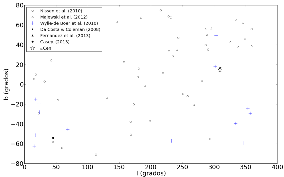
Figura 2.7: Izquierda: Distribución espacial en el plano (l,b) , de todas las estrellas asociadas a Omega Centauri basado en lo similar de sus propiedades químicas y cinemáticas. Cada símbolo corresponde al sondeo realizado por diferentes autores.
